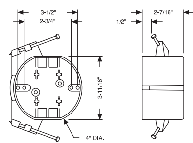
CAT. NOS. 7823, 7824, 9824
