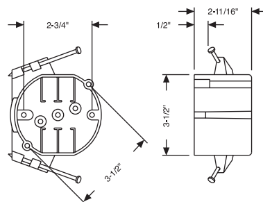
CAT. NOS. 7119, 7919
