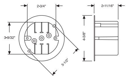
CAT. NOs. 7122, 7922
